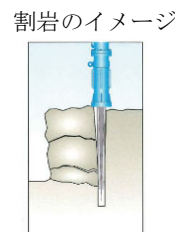
ビッカー(くさび状のセリ矢)を使用して油圧の力で岩を割ります
