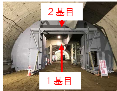
仮設備工（防音、飛石対策） 防音扉設置
