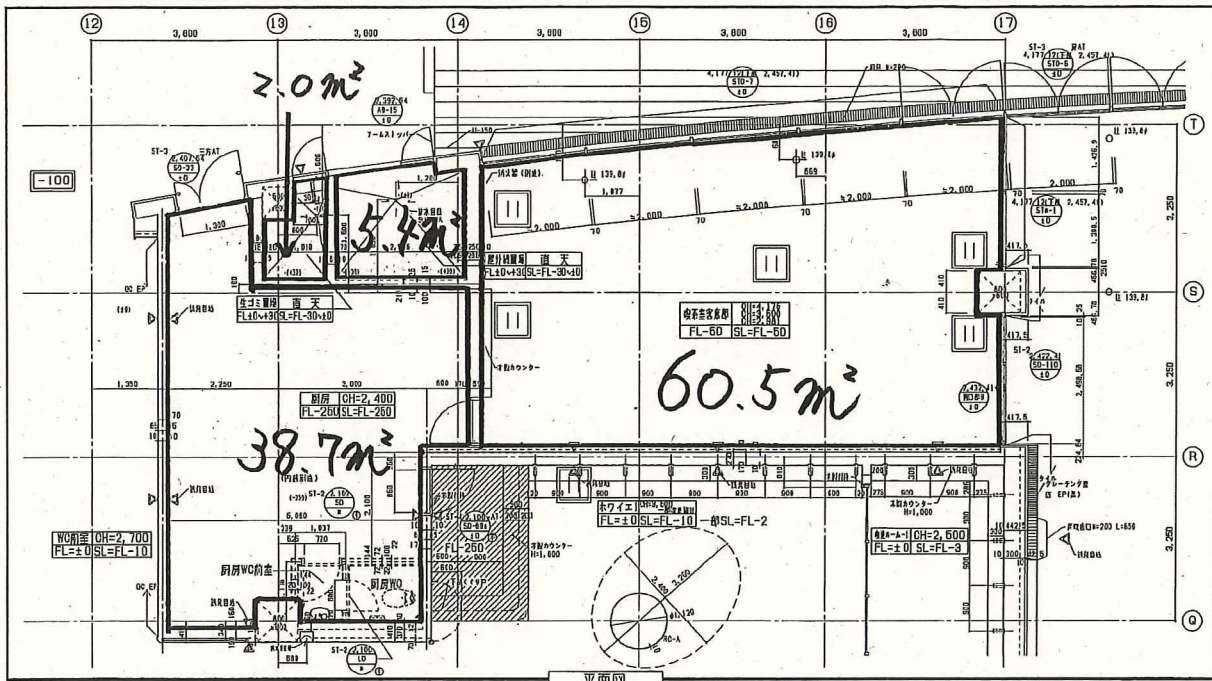
平面図
