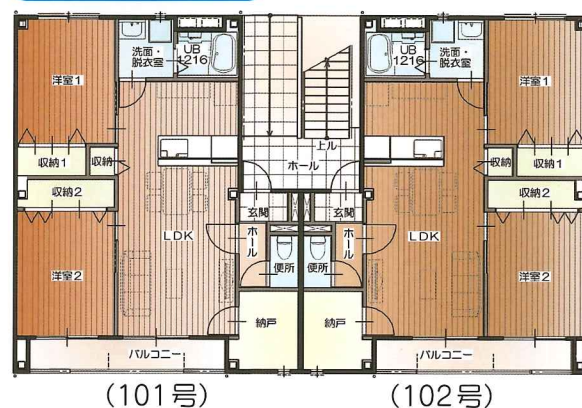
間取り図(1階)
