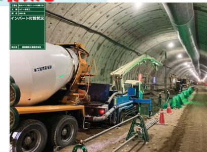
インパルトコンクリート打設状況
