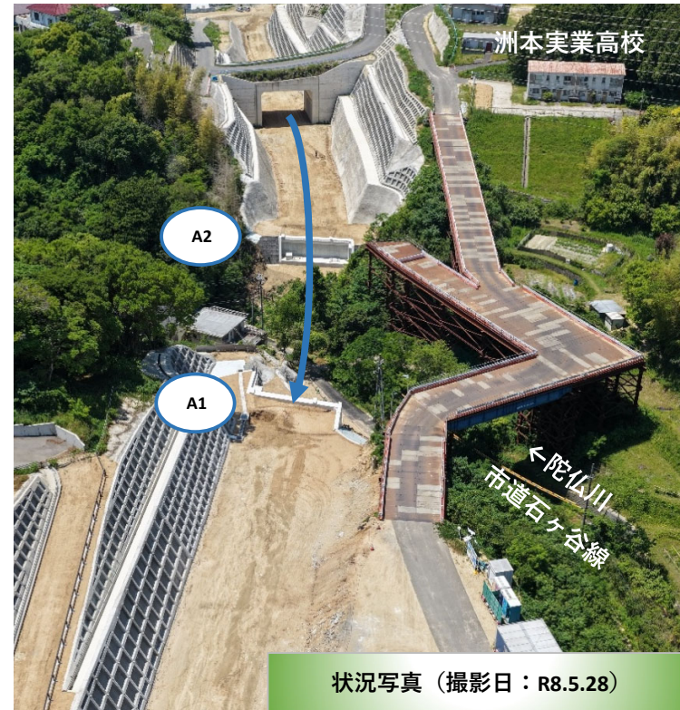
A2橋台付近 仮設工（ヤード整備中）
