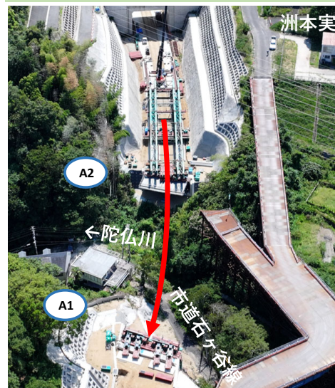
A1橋台付近 仮設工（組立完了）
