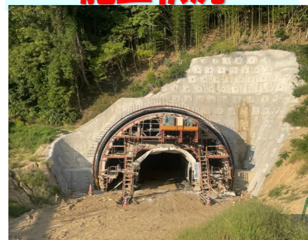
終点側(宇山)坑門工施工状況
